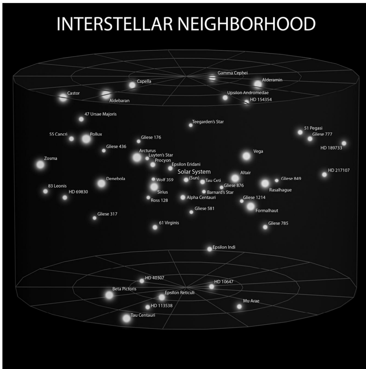
Sluneční mezihvězdné susedství
